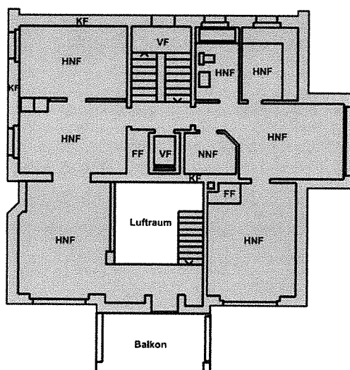
Grundriss 1. Obergeschoss:
